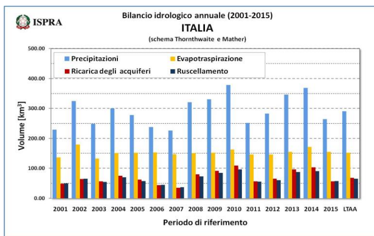
Fig. 21 - Bilancio idrologico annuale (2001-2015)
