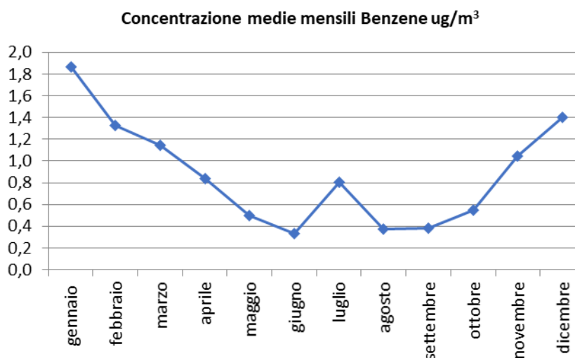
Figura 8 - Andamento delle concentrazioni medie mensili di Benzene – 2020
