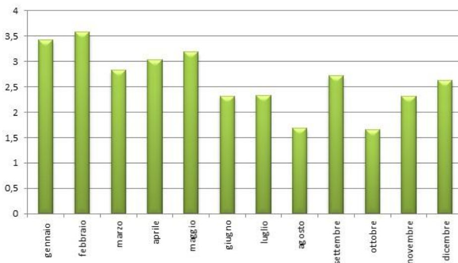
Figura 23 – Velocità del vento medie mensili registrate (m/s) – 2020
