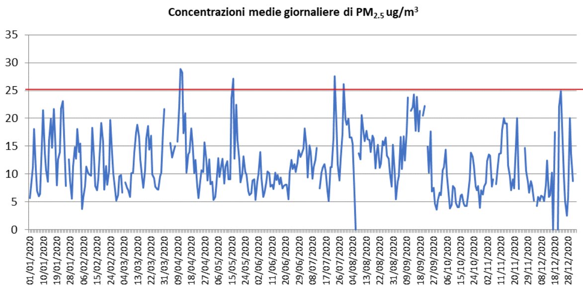
Figura 6 - Andamento delle concentrazioni medie giornaliere di PM 2.5 - 2020
