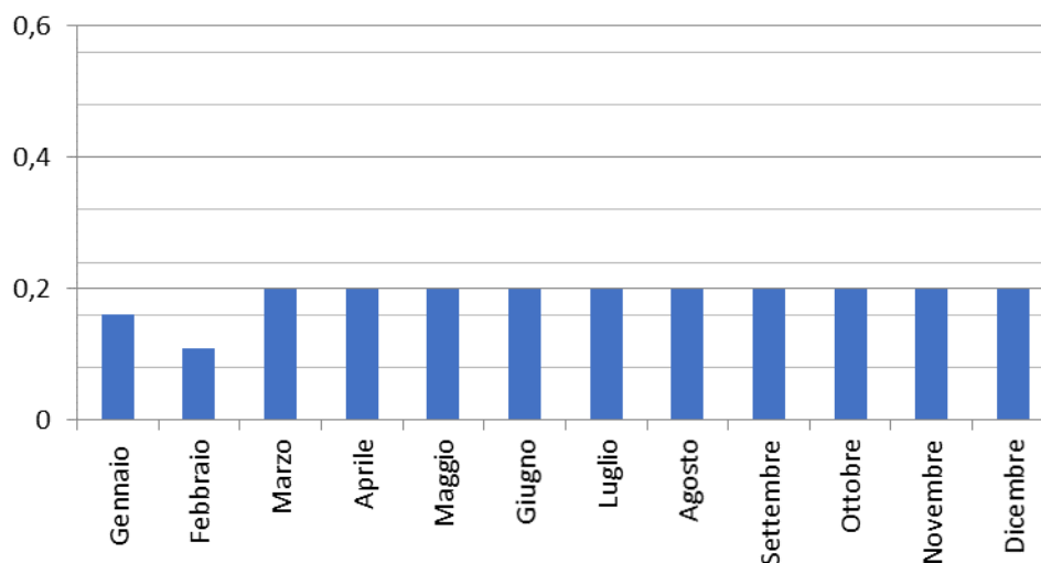
Figura 10 - Andamento delle concentrazioni medie mensili di ARSENICO in ng/m 3 nel periodo considerato - 2020
