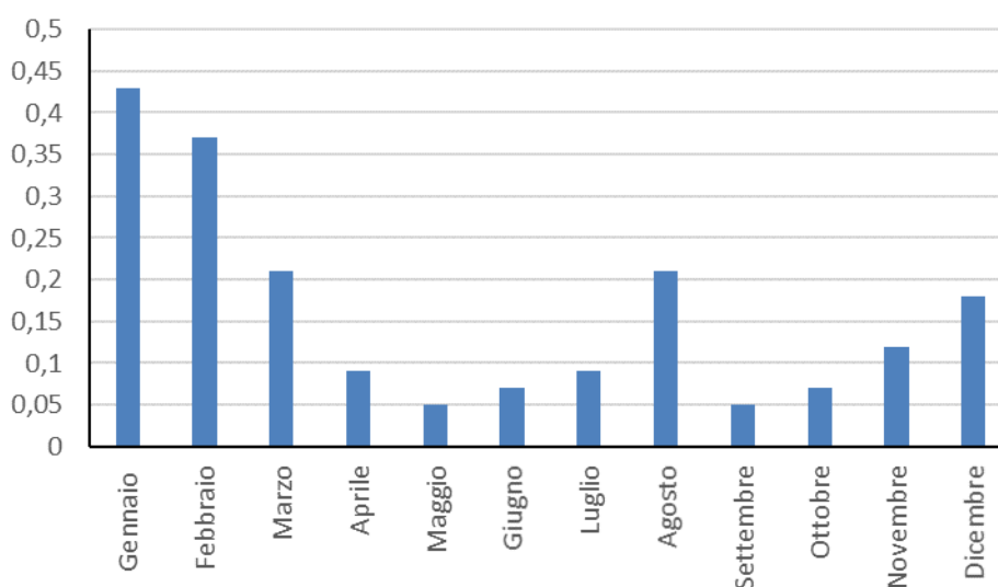
Figura 19 - Andamento delle concentrazioni medie mensili di Benzo[a]pirene nel periodo considerato – 2020
