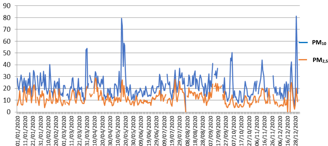
Figura 7 - Andamento delle concentrazioni medie giornaliere di PM 10 e PM 2.5 – 2020
