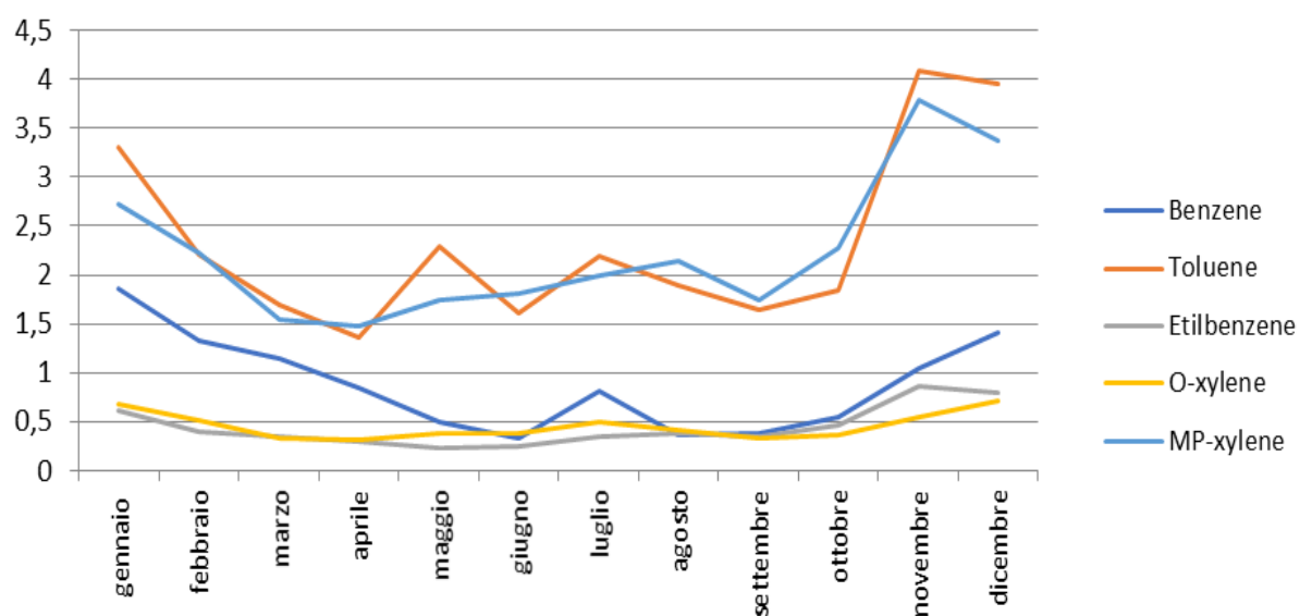
Figura 9 - Andamento delle concentrazioni medie mensili di BTEX - 2020
