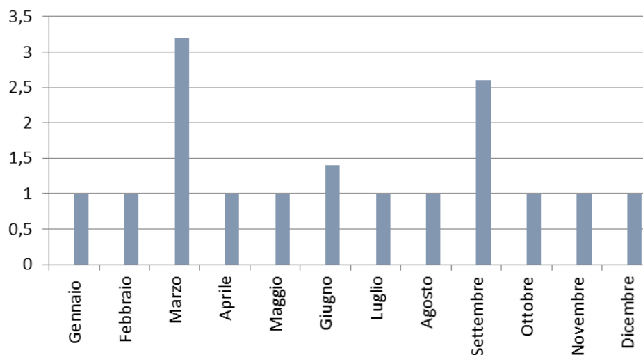
Figura 14 - Andamento delle concentrazioni medie mensili di Nichel nel periodo considerato - 2020
