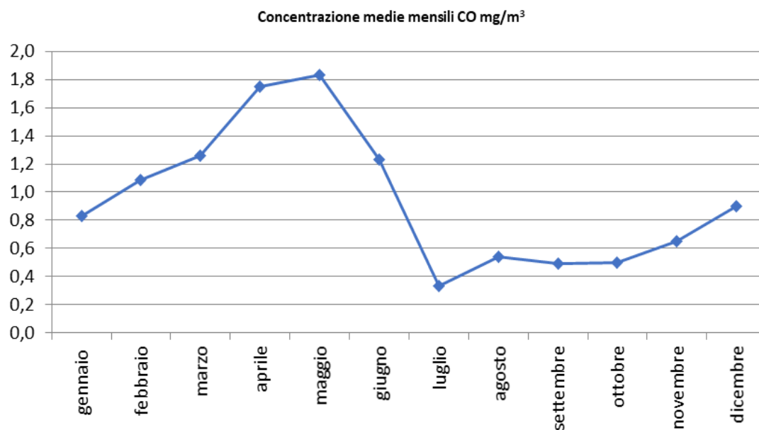
Figura 1 - Andamento delle concentrazioni medie mensili di CO – 2020
