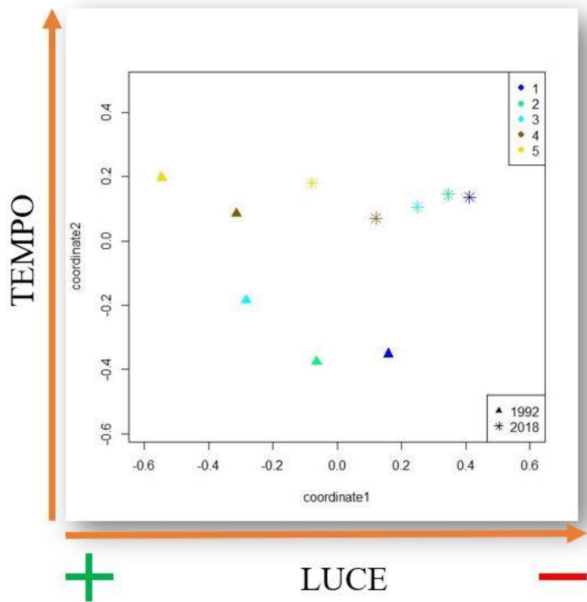
GRAFICO 3-4: nMDS delle stazioni topografiche individuate all'entrata della Grotta Azzurra di Capo Palinuro e interpretazione degli assi.
