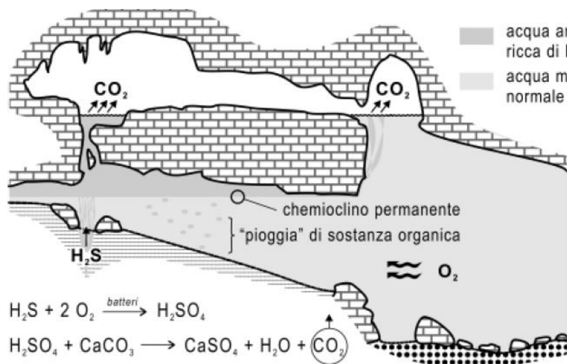
Figura 16: Schema ipotetico del metabolismo solfo-batterico e del significato della produzione chemiolitoautotrofa nella Grotta Azzurra di Capo Palinuro (da Bianchi et al., 1996, modificato).
