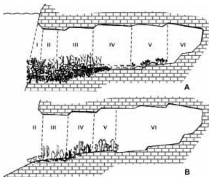
Figura 9: Zone biotiche in una grotta marina superficiale, situata a 1-5 m di profondità (A), ed in una profonda, a 15-40 m (B) (Da Riedl, 1966, modificato).
