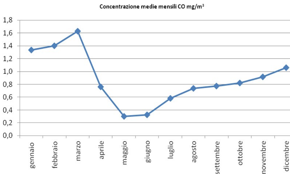
Figura 1 - Andamento delle concentrazioni medie mensili di CO – 2018
