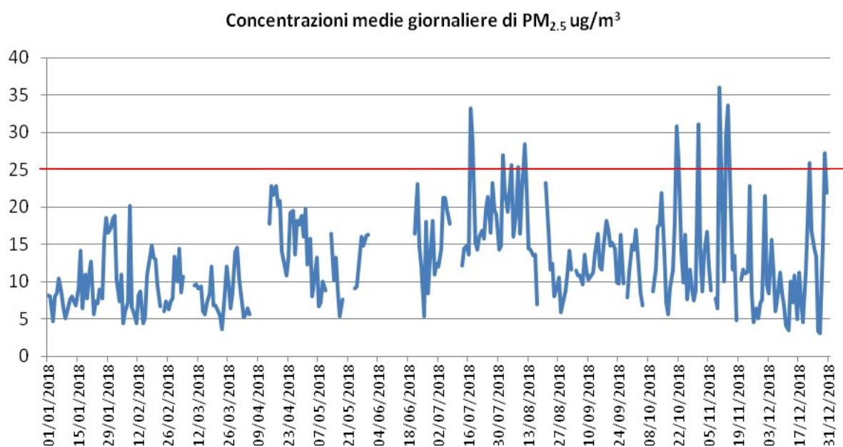
Figura 6 - Andamento delle concentrazioni medie giornaliere di PM 2,5 - 2018
