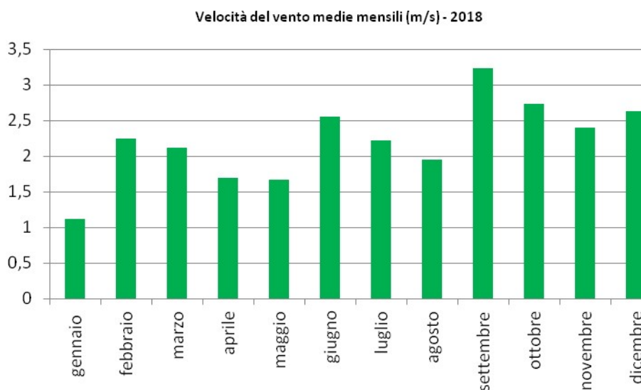
Figura 23 – Velocità del vento medie mensili registrate (m/s) – 2018
