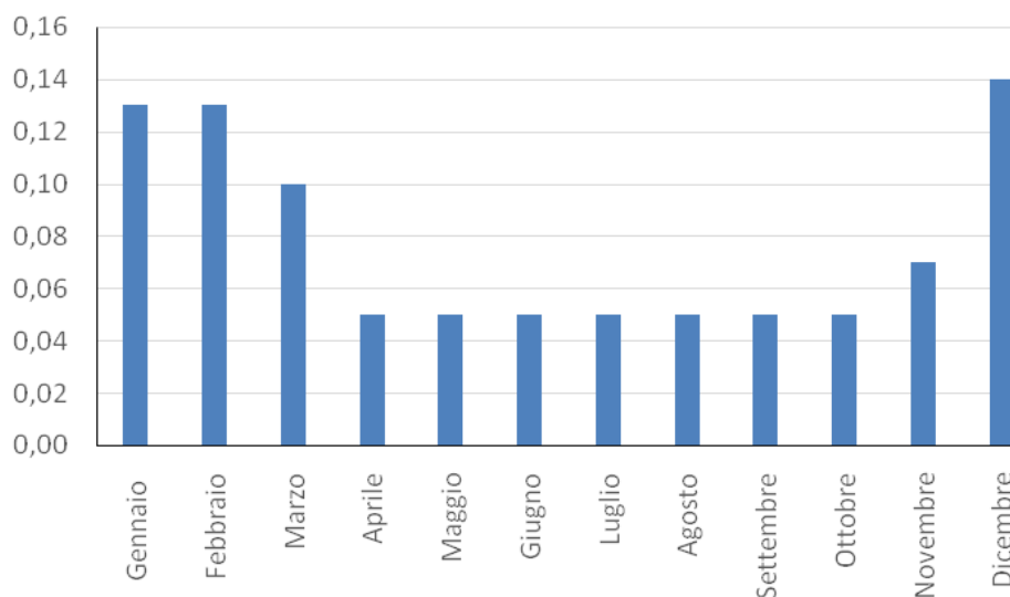
Figura 19 - Andamento delle concentrazioni medie mensili di Benzo[a]pirene nel periodo considerato - 2017
