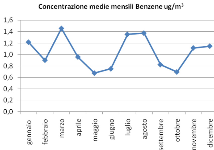
Figura 8 - Andamento delle concentrazioni medie mensili di Benzene – 2017
