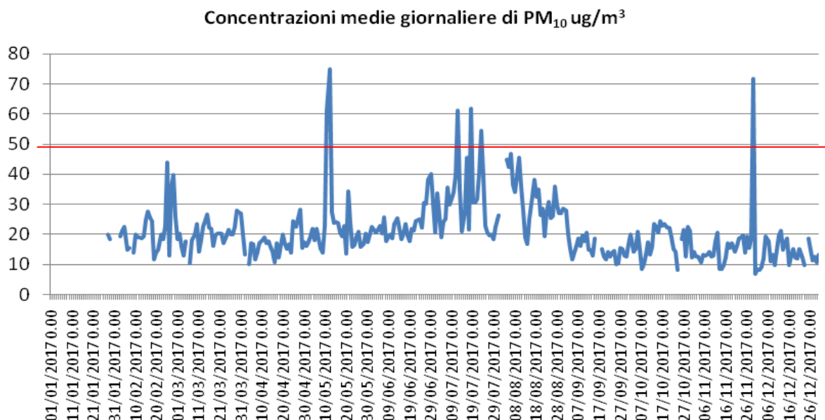
Figura 5 - Andamento delle concentrazioni medie giornaliere di PM 10 – 2017
