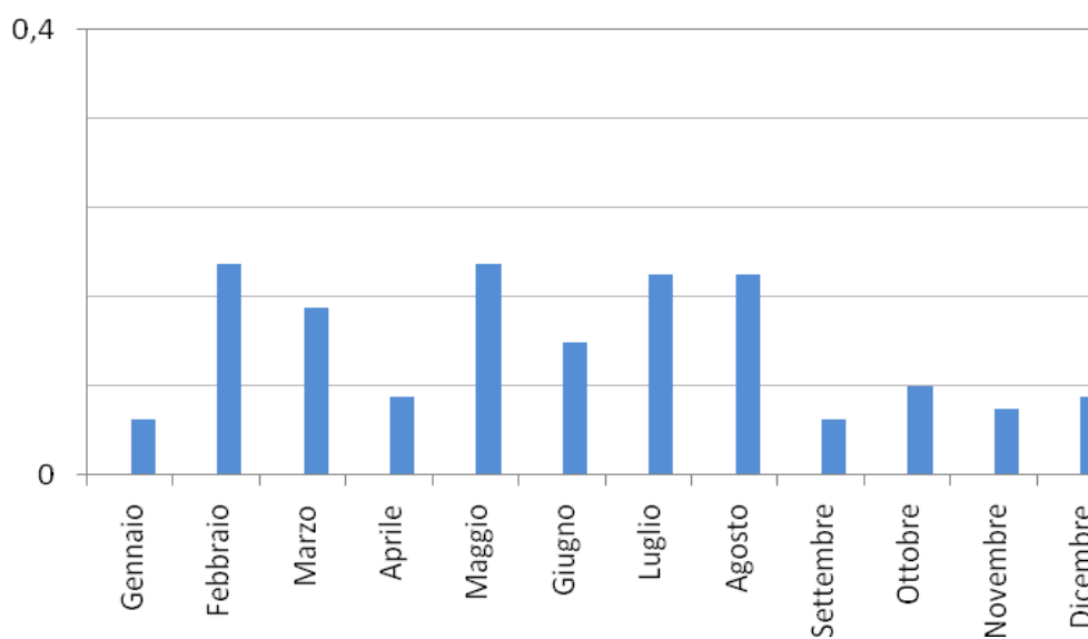
Figura 12 - Andamento delle concentrazioni medie mensili di Cadmio nel periodo considerato - 2017
