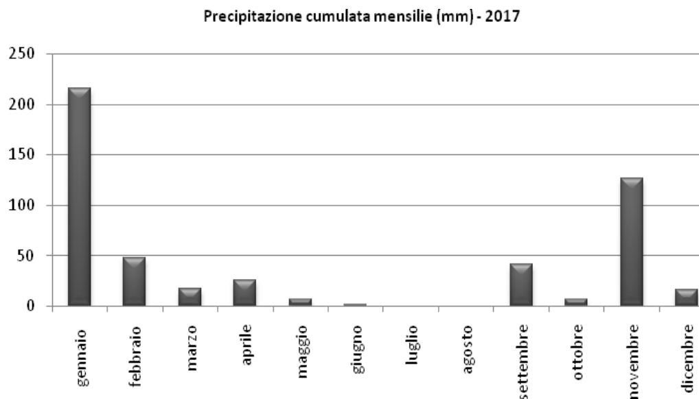
Figura 21 - Precipitazione cumulata mensile registrata (mm) – 2017
