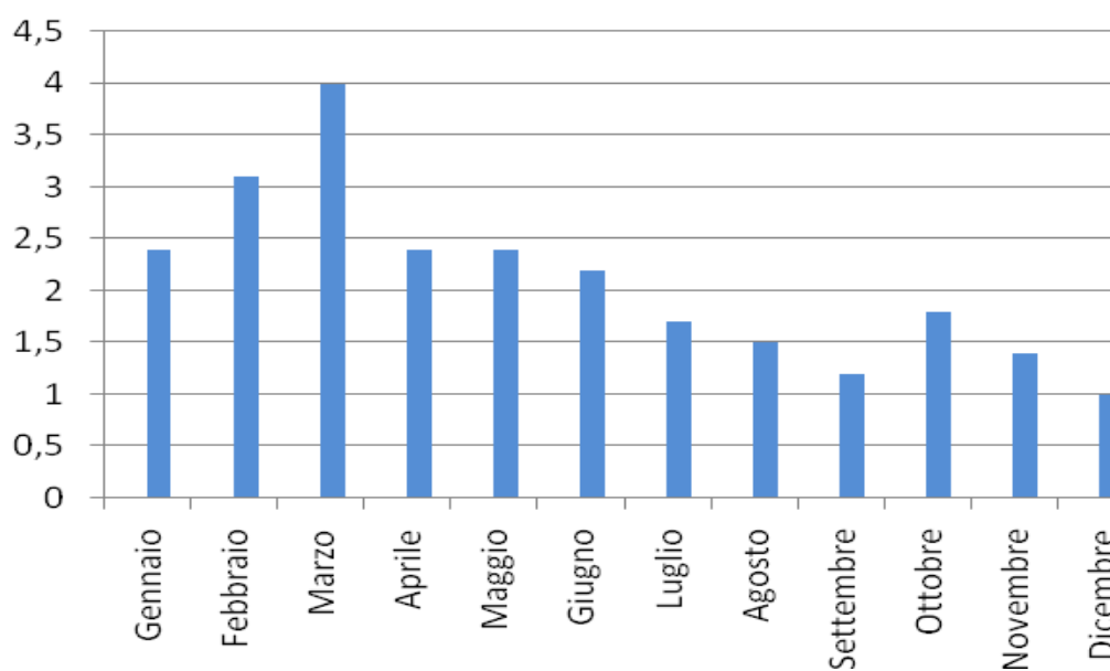
Figura 14 - Andamento delle concentrazioni medie mensili di Nichel nel periodo considerato - 2017
