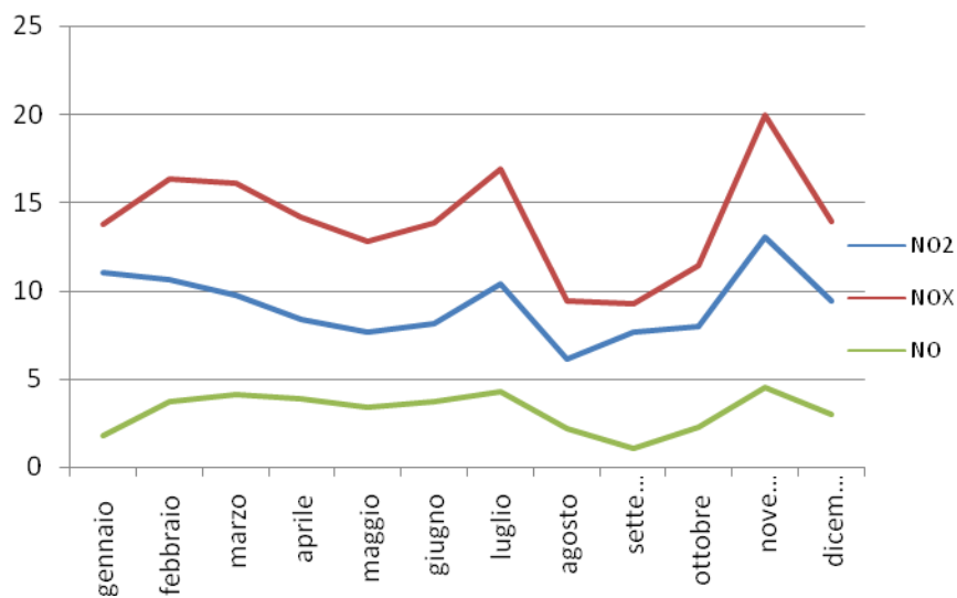
Figura 4 - Andamento delle concentrazioni medie mensili di NO 2 - NO x - NO - 2017
