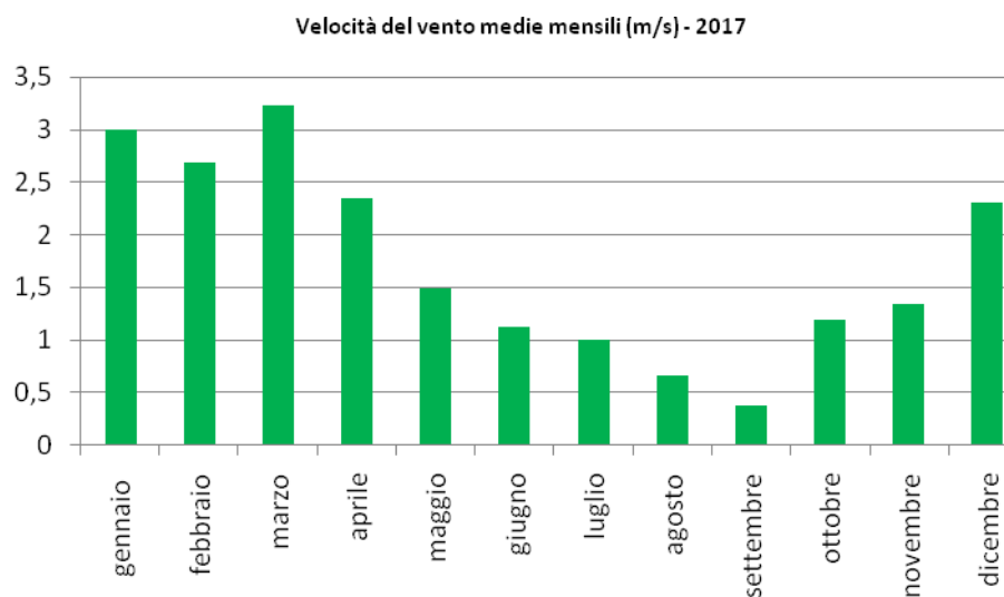
Figura 23 – Velocità del vento medie mensili registrate (m/s) – 2017
