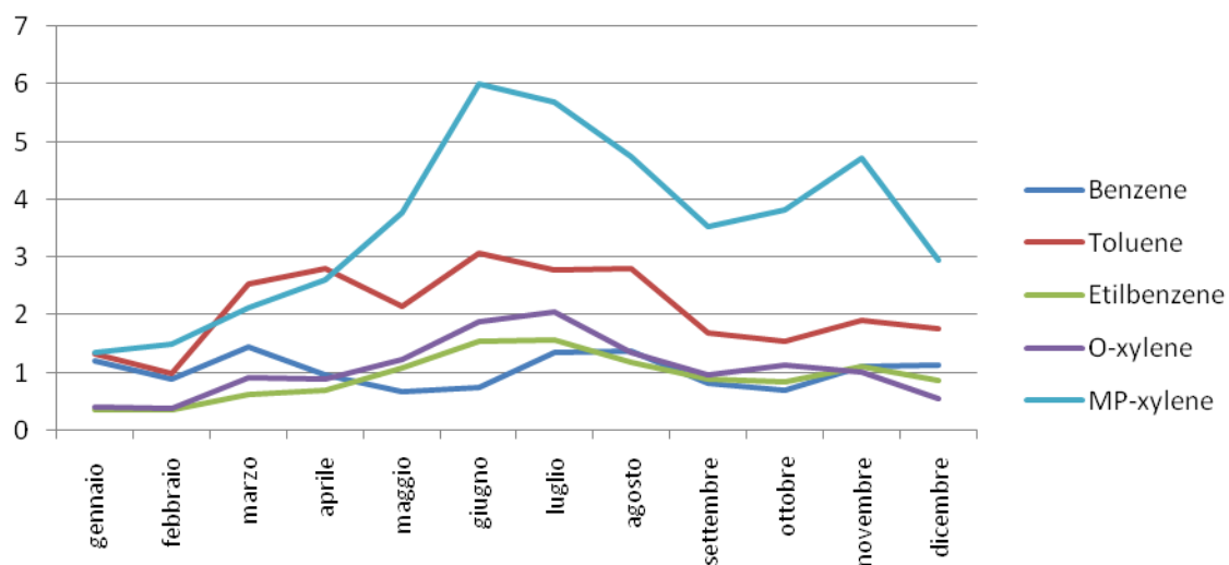
Figura 9 - Andamento delle concentrazioni medie mensili di BTEX - 2017
