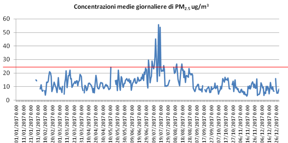
Figura 6 - Andamento delle concentrazioni medie giornaliere di PM 2.5 - 2017
