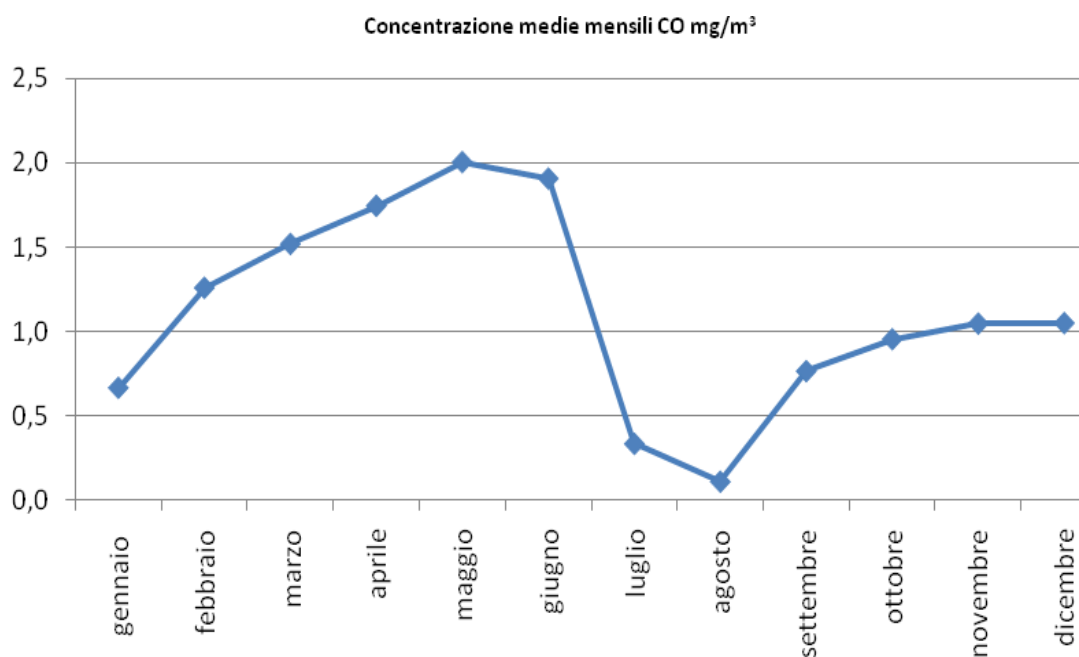
Figura 1 - Andamento delle concentrazioni medie mensili di CO – 2017
