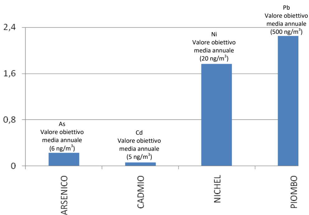
Figura 18 - Andamento delle concentrazioni annuali dei metalli (ng/m 3 ) con evidenza del valore obiettivo - 2017 -
