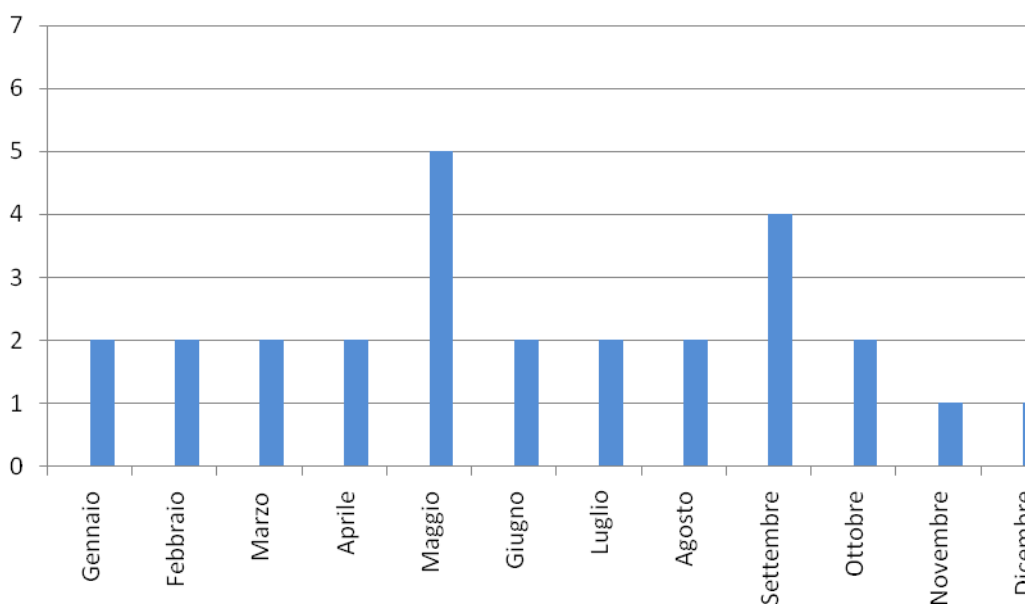
Figura 16 - Andamento delle concentrazioni medie mensili di Piombo nel periodo considerato – 2017
