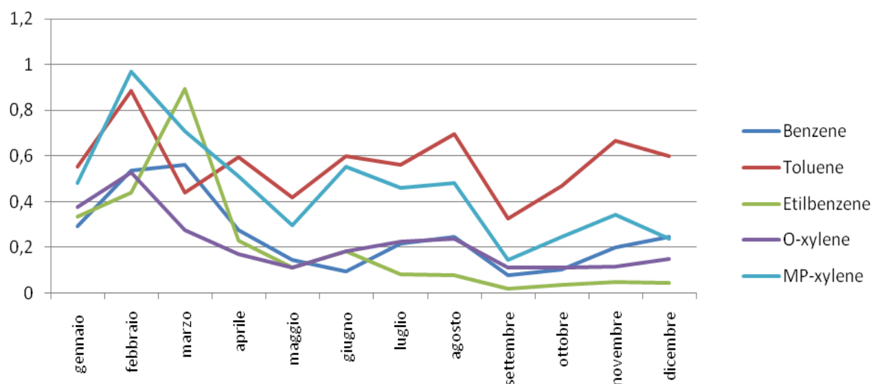
Figura 9 - Andamento delle concentrazioni medie mensili di BTEX - 2017
