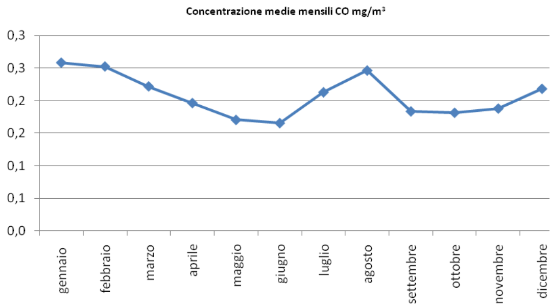
Figura 1 - Andamento delle concentrazioni medie mensili di CO – 2017
