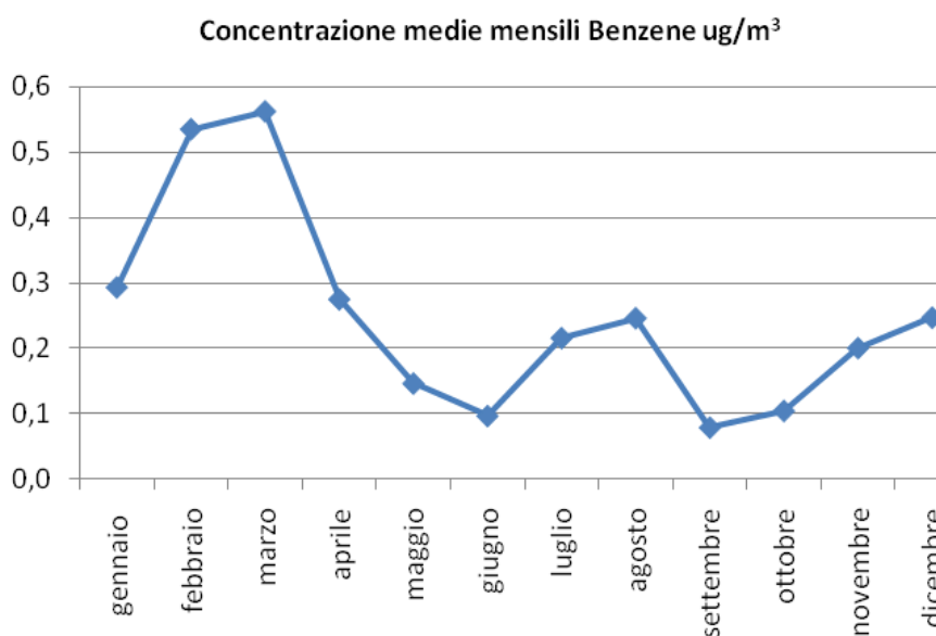
Figura 8 - Andamento delle concentrazioni medie mensili di Benzene – 2017
