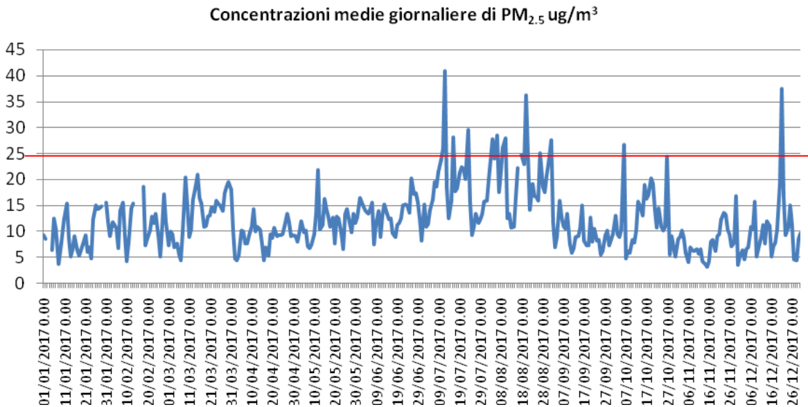
Figura 6 - Andamento delle concentrazioni medie giornaliere di PM 2,5 - 2017
