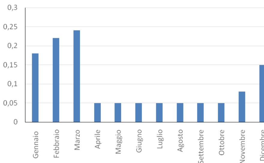
Figura 19 - Andamento delle concentrazioni medie mensili di Benzo[a]pirene nel periodo considerato - 2017
