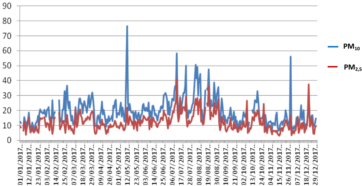
Figura 7 - Andamento delle concentrazioni medie giornaliere di PM 10 e PM 2,5 – 2017
