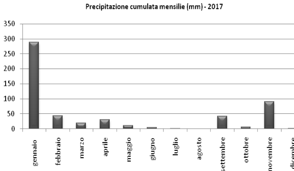
Figura 21 - Precipitazione cumulata mensile registrata (mm) – 2017
