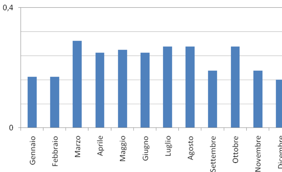
Figura 10 - Andamento delle concentrazioni medie mensili di ARSENICO in ng/m 3 nel periodo considerato - 2017
