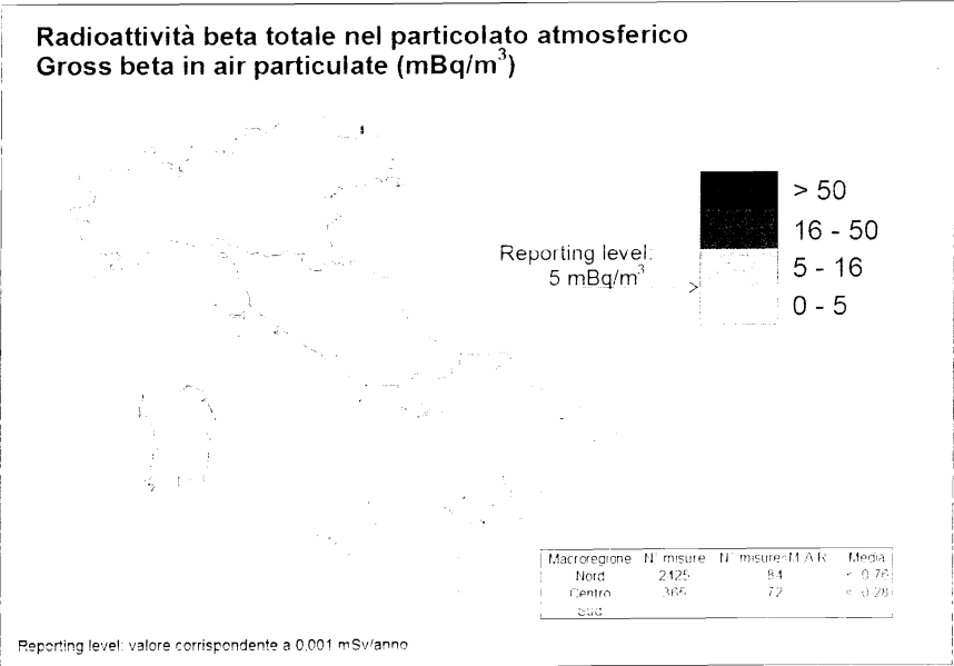
Figura 2 - Radioattività beta totale nel particolato atmosferico – Gross beta in air particulate. (mBq/m³)
