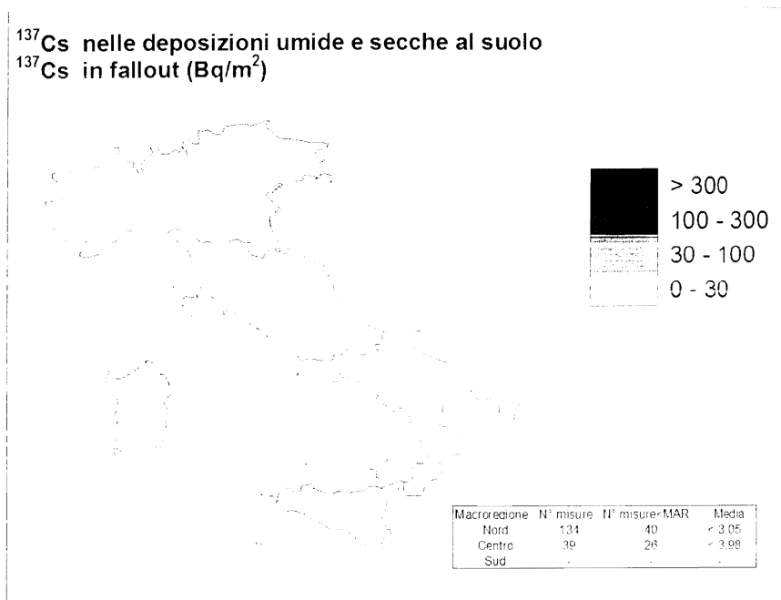
Figura 8 - Concentrazione di ^{137}\text{Cs} nelle deposizioni umide e secche annuali al suolo – ^{137}\text{Cs} in fallout, ( \text{Bq/m}^2 )
