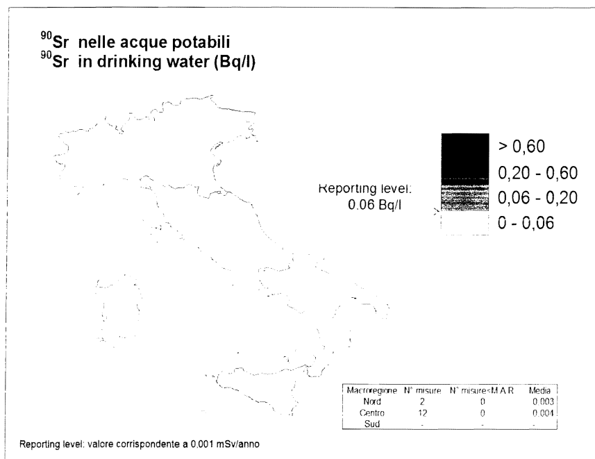
Figura 15 - Concentrazione di 90 Sr nelle acque potabili – 90 Sr in drinking water. (Bq/l)
