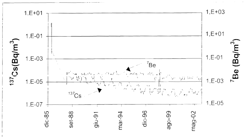
Figura 6 - Andamenti delle concentrazioni di ^{137}\text{Cs} e ^7\text{Be} della stazione di prelievo della rete RESORAD di Milano (ARPA Lombardia) – Trends of ^{137}\text{Cs} and ^7\text{Be} obtained at the sampling point of RESORAD network of Milano (ARPA Lombardia)
