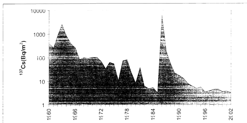
Figura 9 - Andamento del ^{137}\text{Cs} nelle deposizioni umide e secche annuali al suolo – Trend of ^{137}\text{Cs} in fallout, ( \text{Bq/m}^2 )
