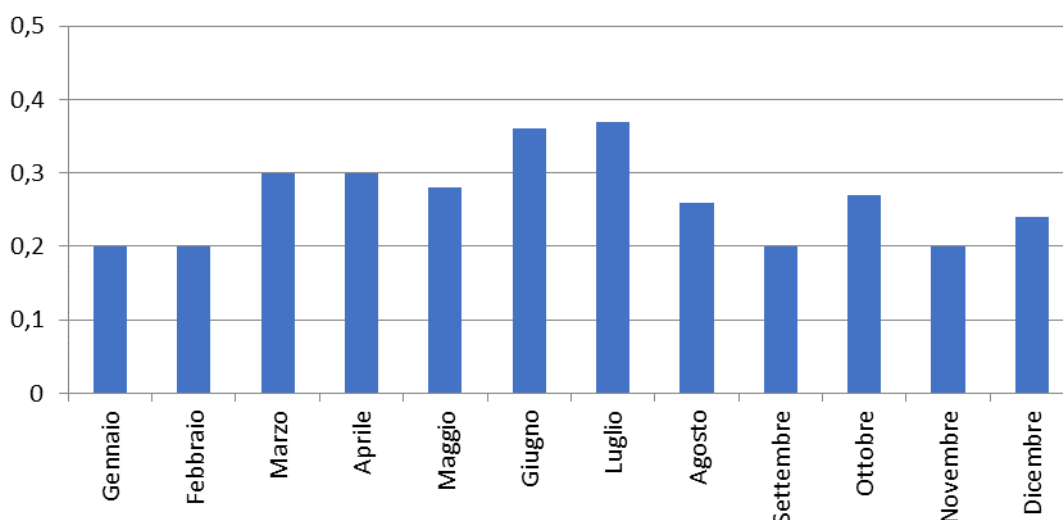
Figura 10 - Andamento delle concentrazioni medie mensili di ARSENICO in ng/m 3 nel periodo considerato - 2022
