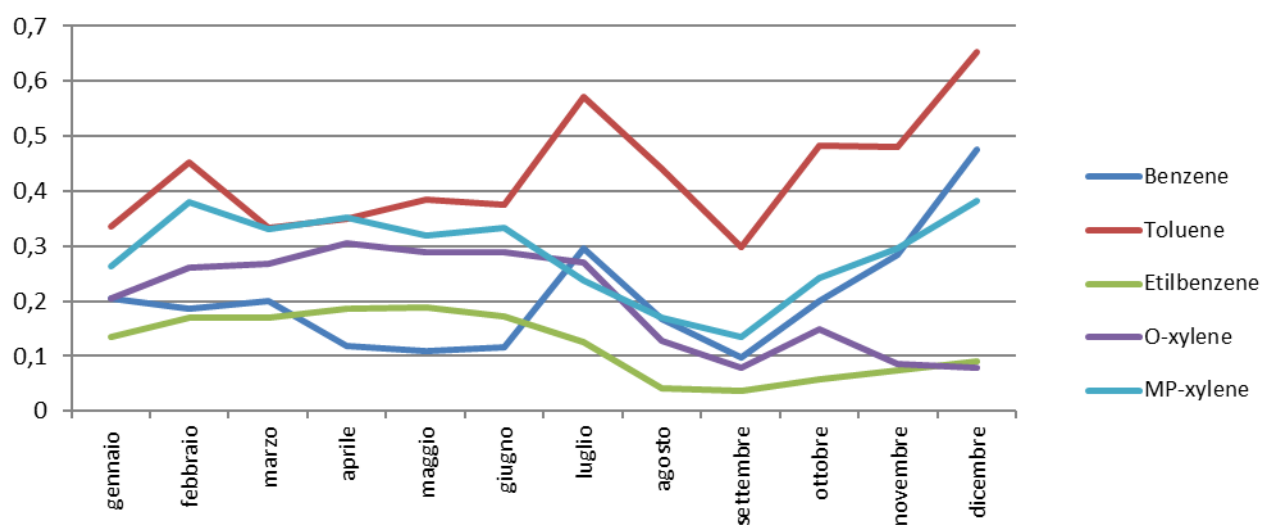
Figura 9 - Andamento delle concentrazioni medie mensili di BTEX - 2022
