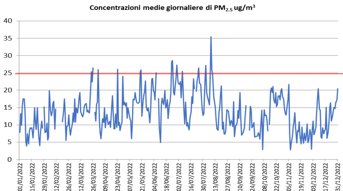
Figura 6 - Andamento delle concentrazioni medie giornaliere di PM 2.5 - 2022
