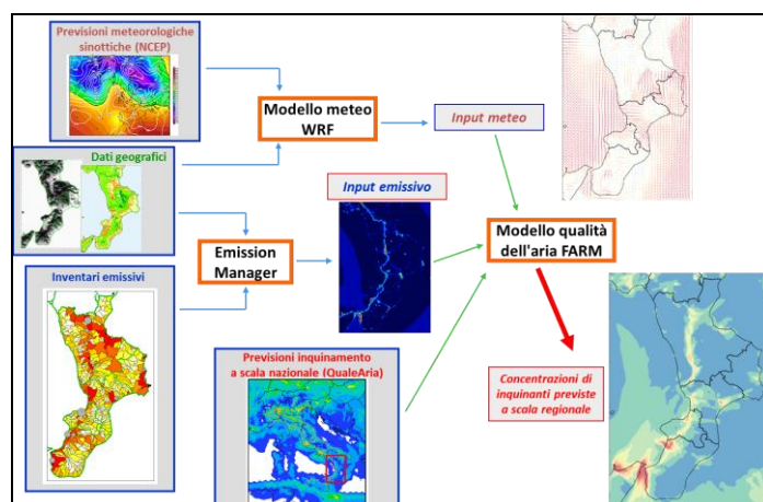
Figura 21: sistema modellistico utilizzato per la Valutazione della Qualità dell’Aria nella Regione Calabria
