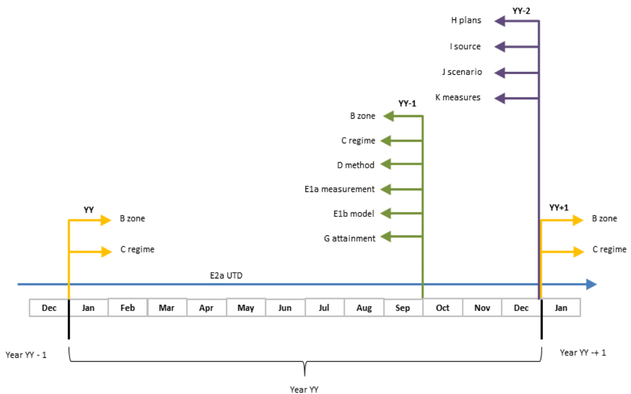
Figura 18: Ciclo di reporting europeo.
