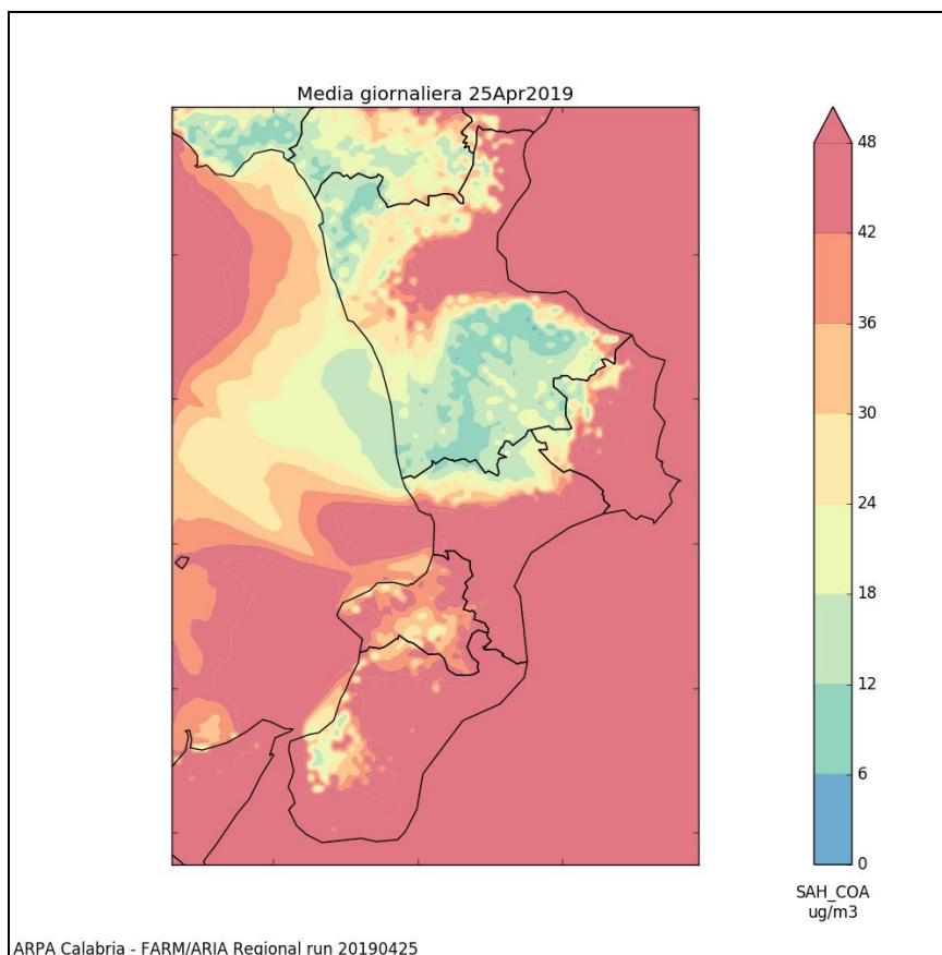
Figura 24: campi di concentrazione medi giornalieri derivante da post-elaborazione con contributo di polveri sahariane fini
