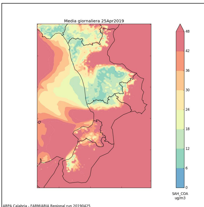
Figura 23: campi di concentrazione medi giornalieri derivante da post-elaborazione con contributo di polveri sahariane grossolane
